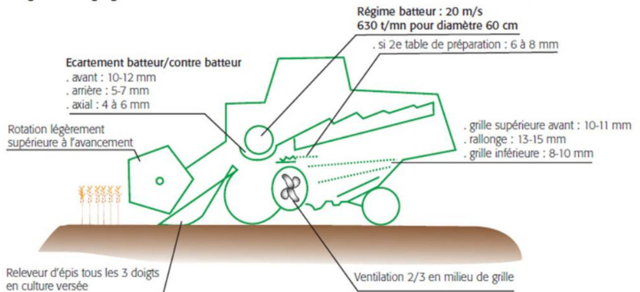
Figure 1 : Réglages de base de la moissonneuse-batteuse – vitesse d'avancement de 4 à 6 km/h
